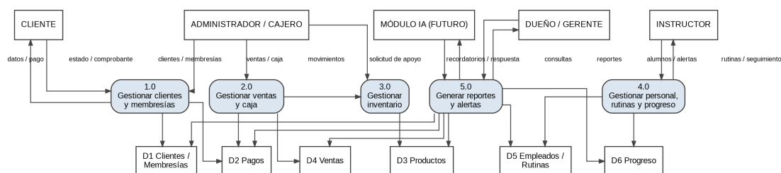
Figura 4: DFD Nivel 1 – Sistema de Gestión FabroGym
