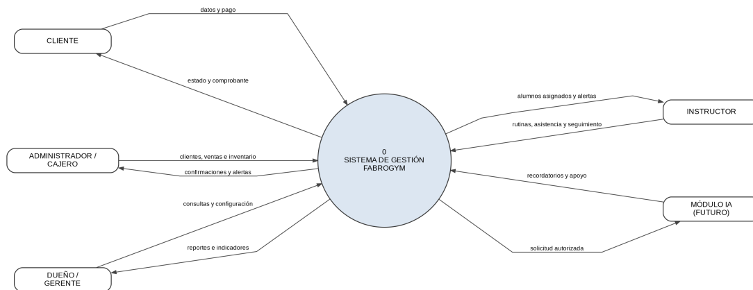
Figura 3: Diagrama de contexto (DFD Nivel 0) – Sistema de Gestión FabroGym
