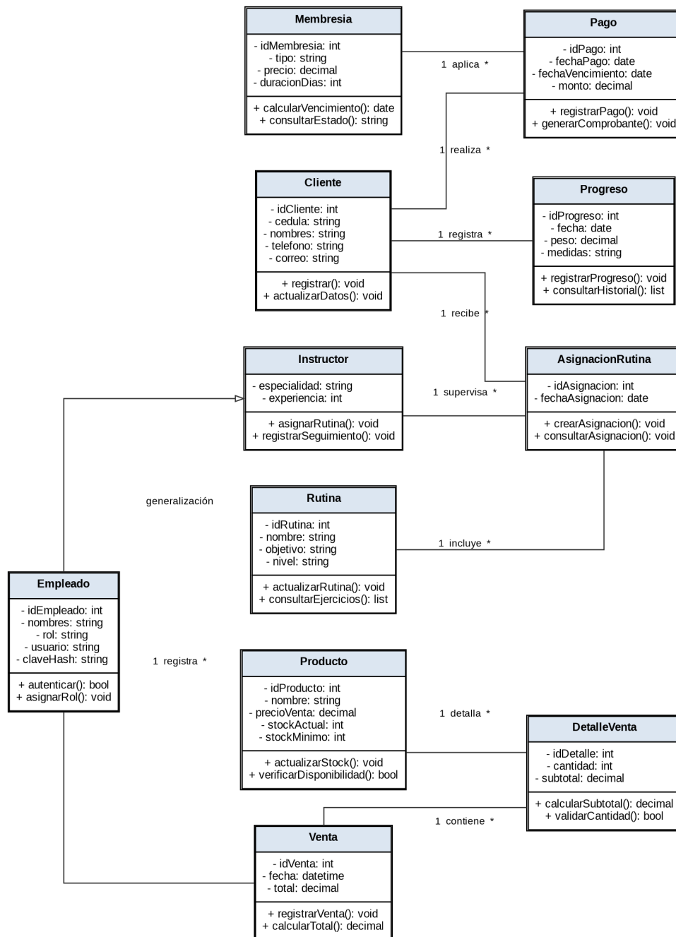
Figura 2: Diagrama de clases UML – Sistema FabroGym
